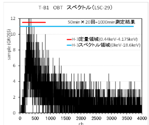
トリチウムのベータ線スペクトルの例
