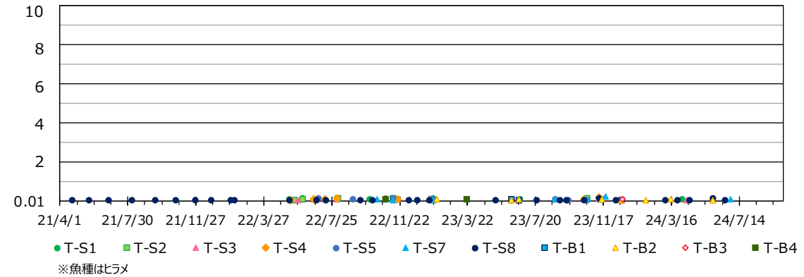
(Ba/L) 魚類 トリチウム濃度 (組織自由水型) (線形グラフ 最小値 0.01 Bq/L)
