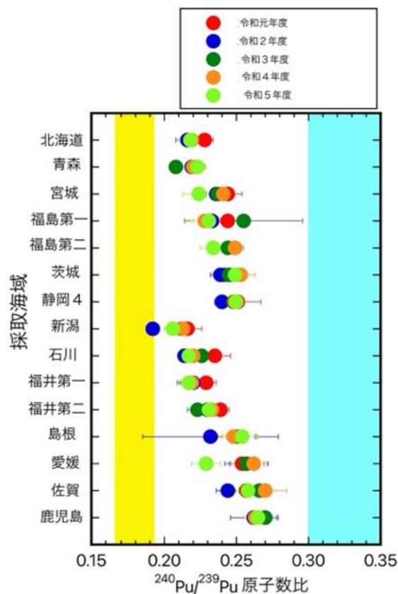
図1-2-3-1-2 発電所海域で採取した海底土に含まれるプルトニウムの ^{240}\text{Pu}/^{239}\text{Pu} 原子数比 (赤色、青色、濃緑色、オレンジ色及び淡緑色は、それぞれ、令和元(平成31)年度、令和2年度、令和3年度、令和4年度及び令和5年度の原子数比を示す。黄色及び水色の網掛けは、それぞれ、グローバルフォールアウト比及び太平洋核実験場起源の局地フォールアウト比を示す。)
