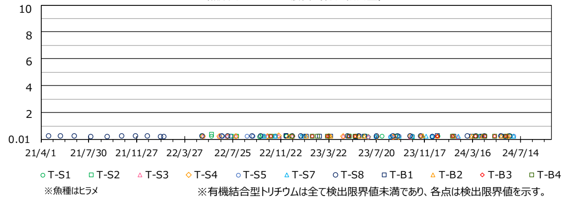
(Ba/L) 魚類 トリチウム濃度 (有機結合型) (線形グラフ 最小値 0.01 Bq/L)
