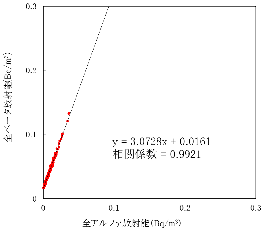
大気浮遊じんの全アルファ・全ベータ放射能の相関図 (MP-1) (令和6年1月～令和6年3月)
