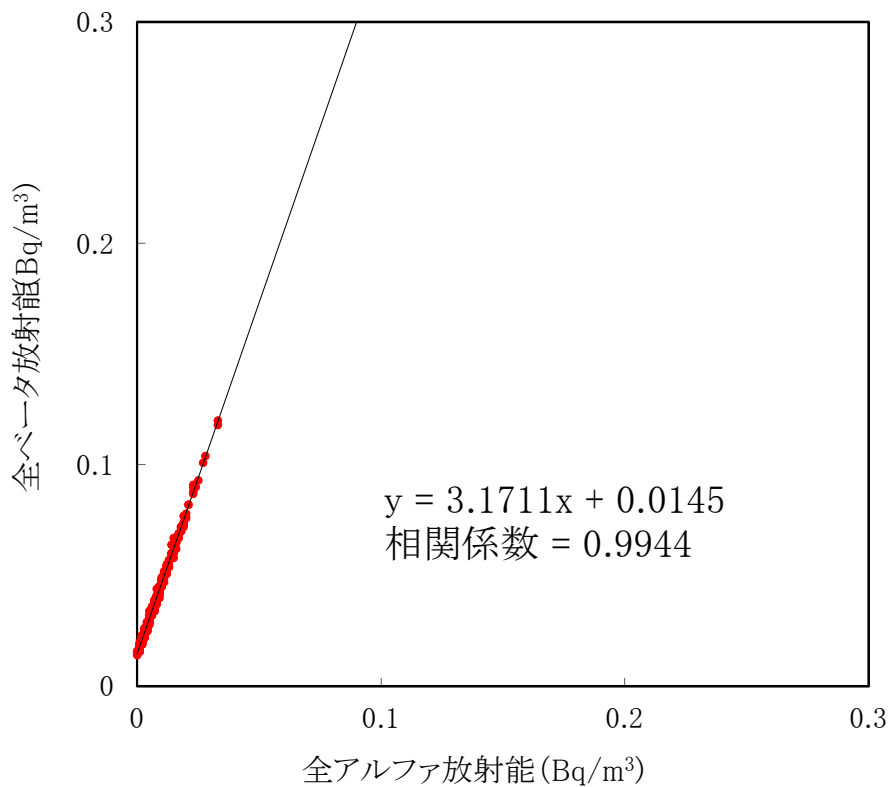
大気浮遊じんの全アルファ・全ベータ放射能の相関図 (MP-7) (令和6年1月～令和6年3月)
