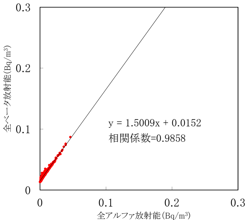
大気浮遊じんの全アルファ・全ベータ放射能の相関図 (MP-8) (令和6年1月～令和6年3月)
