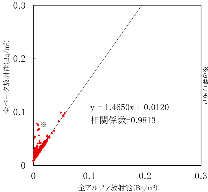
大気浮遊じんの全アルファ・全ベータ放射能の相関図 (MP-3) (令和6年1月～令和6年3月)
