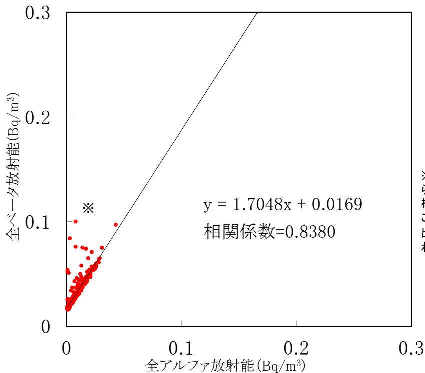
大気浮遊じんの全アルファ・全ベータ放射能の相関図 (MP-8) (令和3年10月～令和3年12月)
