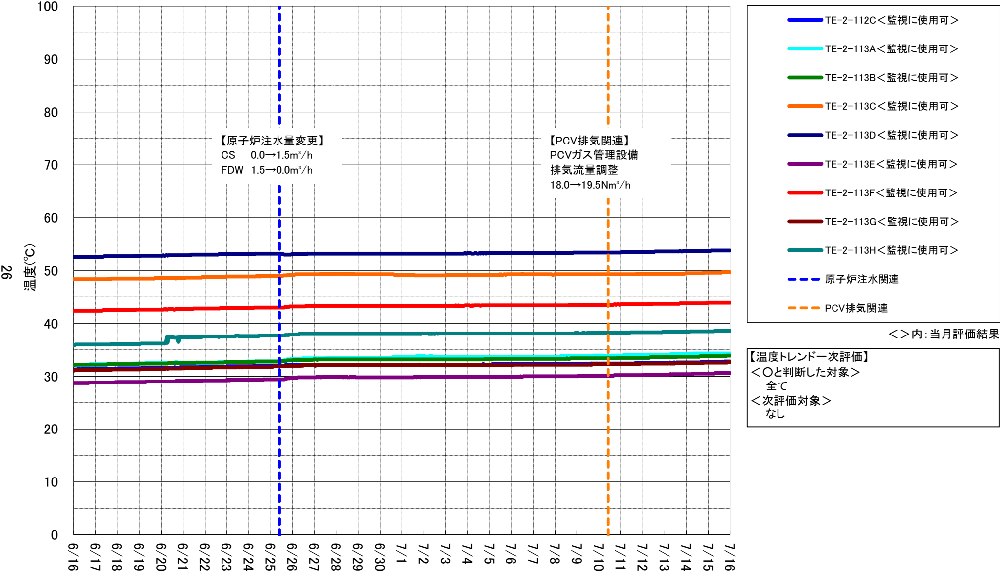
2号機 PCV内温度計①
