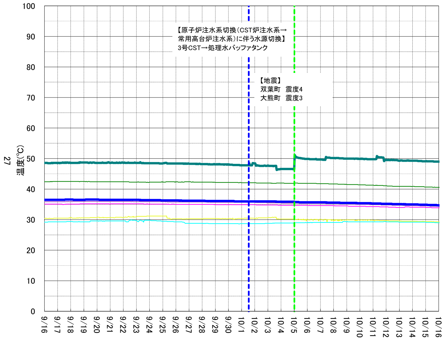
2号機 PCV内温度計②
