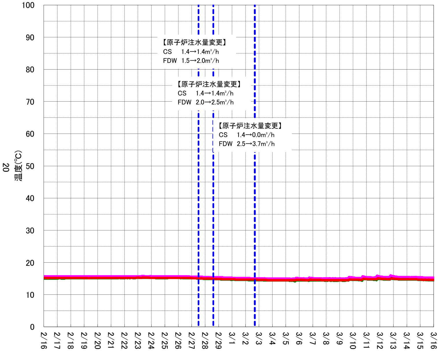
1号機 RPV周辺温度計(下部)
