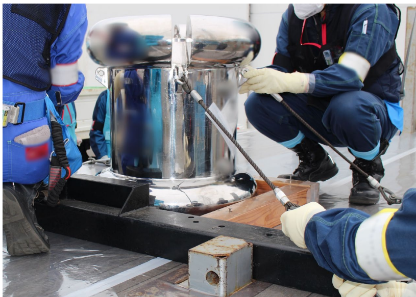
写真1. 構外輸送車両に構外輸送容器を積載する状況 (4月25日午前7時50分頃撮影)
