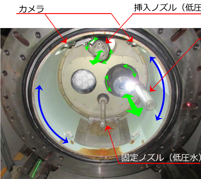
堆積物除去装置（低圧水）X-6ペネ接続断面
