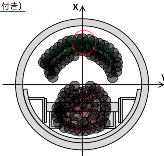
堆積物除去装置（低圧水） 突き崩し実施予定範囲（イメージ）
