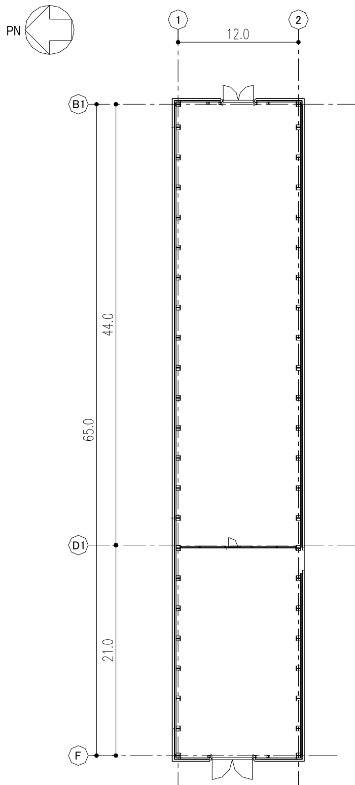
図－１３ 設備棟 建屋平面図 設計 G. L. +0.2 (単位：m)
