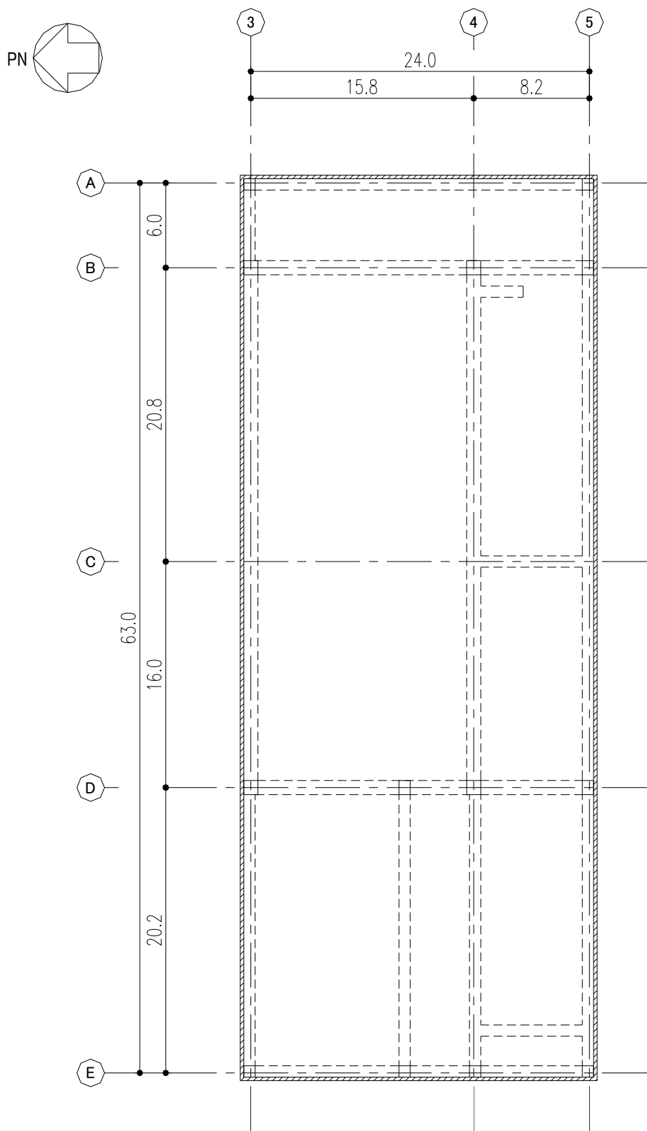
図ー 2 スラッジ棟 屋根平面図（設計 G.L. +11.1）（単位：m）
