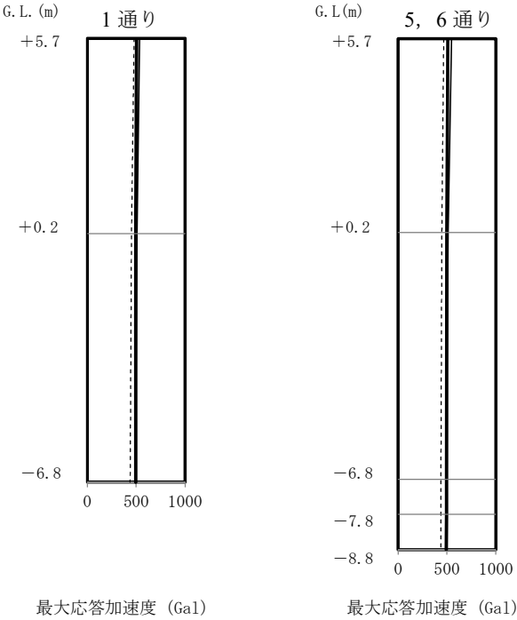
図5-2 最大応答加速度 (EW方向)
