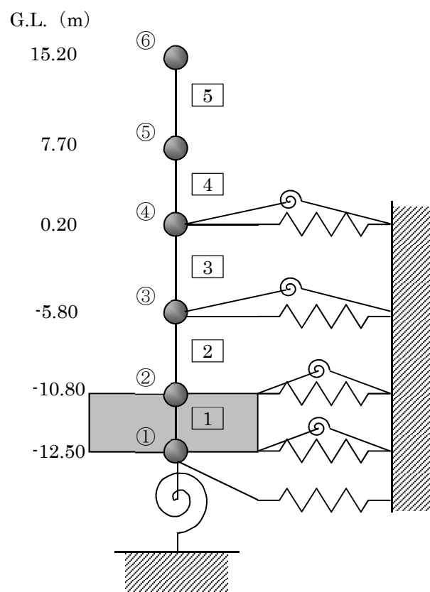
図ー 7 高温焼却炉建屋地震応答解析モデル
