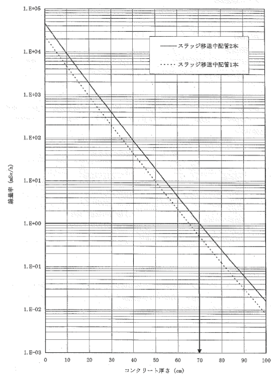
図ー5 配管周りのコンクリート遮へい厚と壁外表面の線量率の関係
