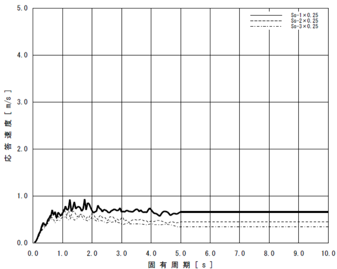
図－３ S P T 建屋 速度応答スペクトル（NS 方向・減衰 0.5%）
