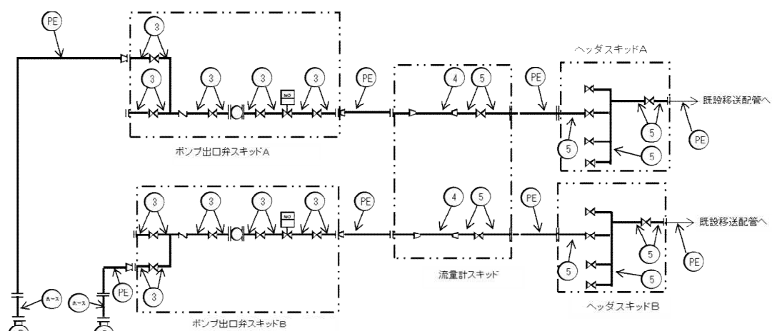
図－1 配管概略図 (5 / 12) (2号機 R/B)
