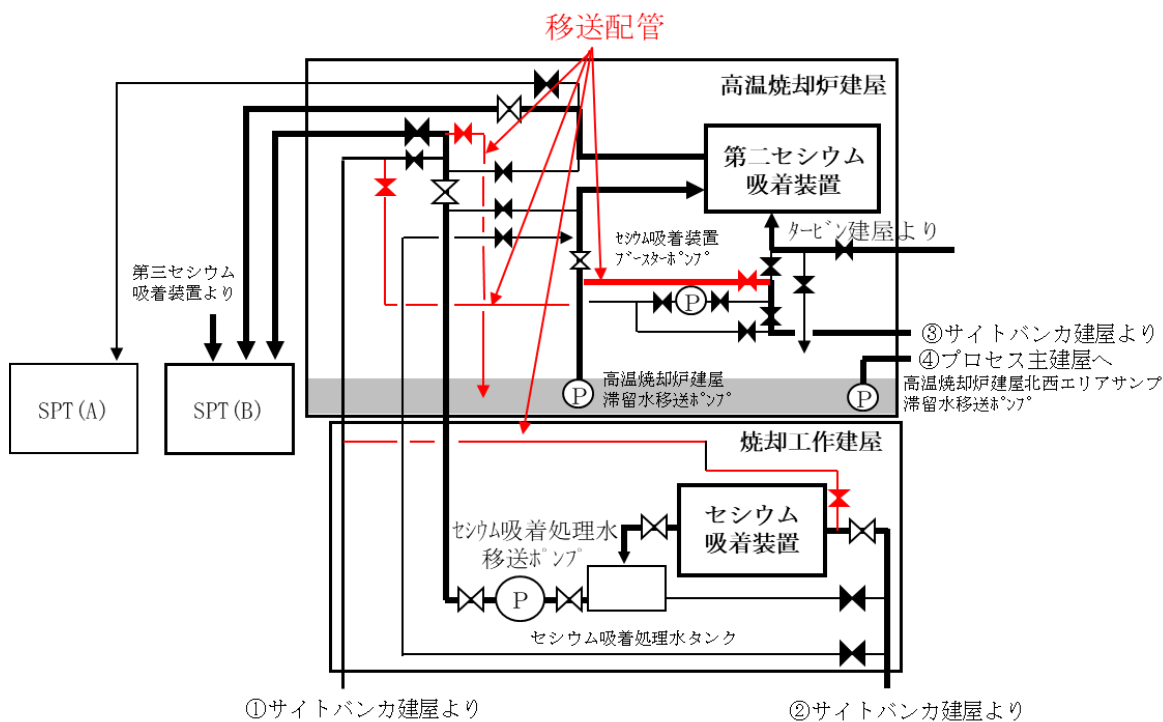
図ー1 処理装置（セシウム吸着装置，第二セシウム吸着装置，第三セシウム吸着装置，除染装置）の系統構成図に対する移送配管の設置範囲
