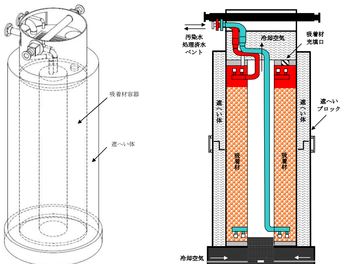
図－１（３／３） 同時吸着塔外形図及び概念図（TYPE-B3）
