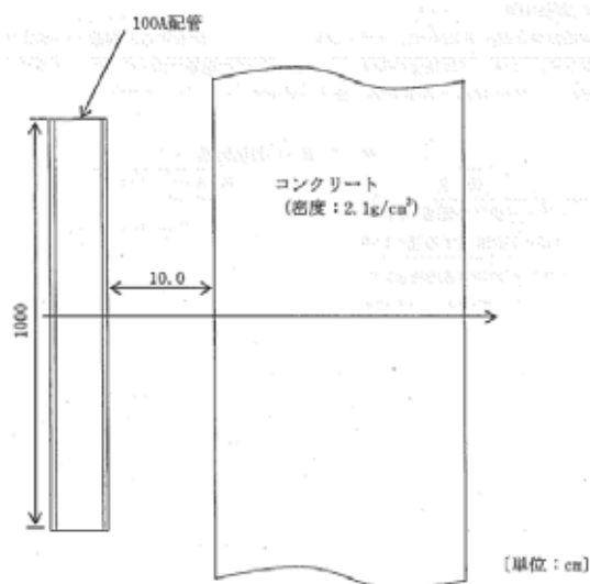
図ー２ 配管遮へい評価モデル
