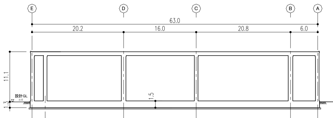
図ー4 スラッジ棟 B-B断面図 (EW 方向) (単位：m)
