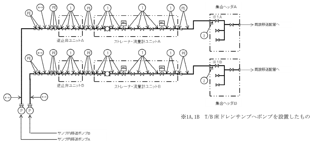
図ー1 配管概略図 (2 / 12)
