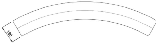
図－８－１ セグメント標準断面図（円周方向）（鉄筋コンクリート造）
