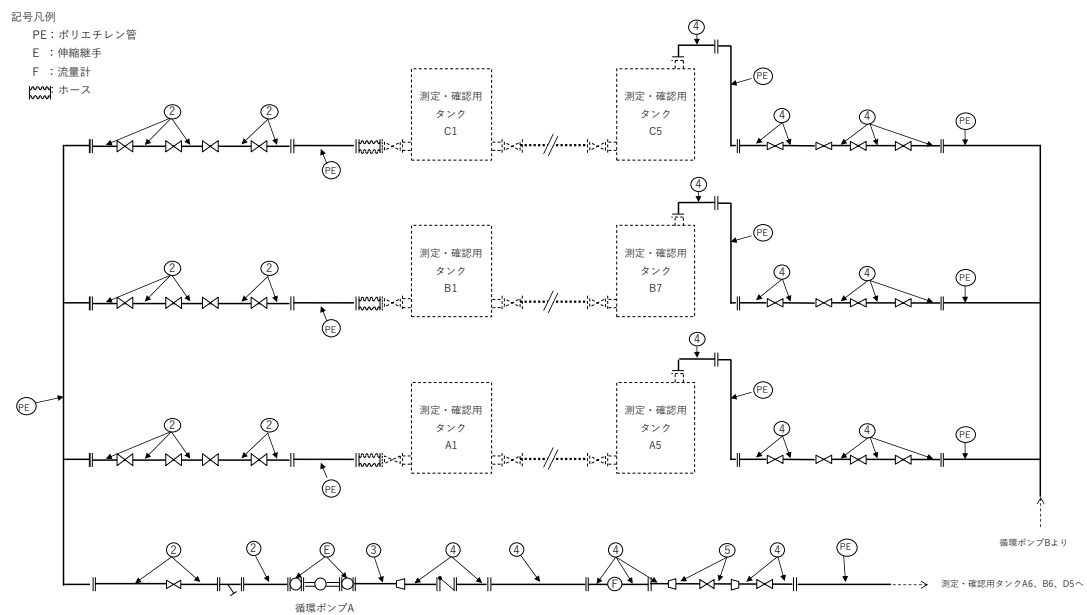
図－２ 配管概略図（２／５） （測定・確認用設備）
