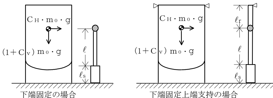
図2-1 固有周期の計算モデル
