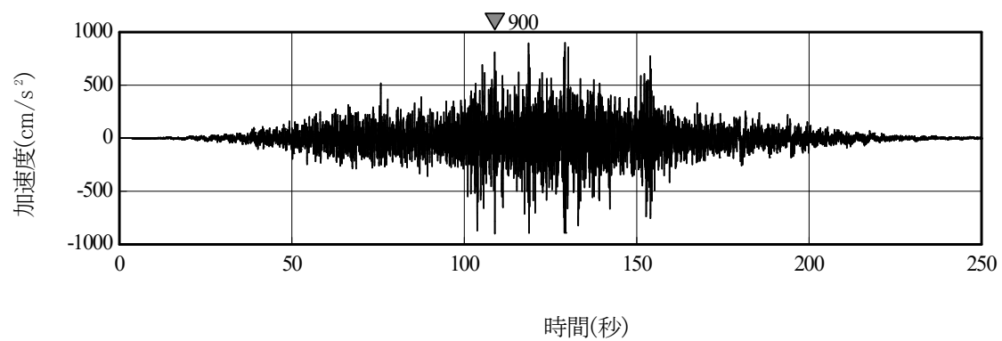
図ー 6 Ss900-1 (水平方向) と組み合わせる模擬地震波
