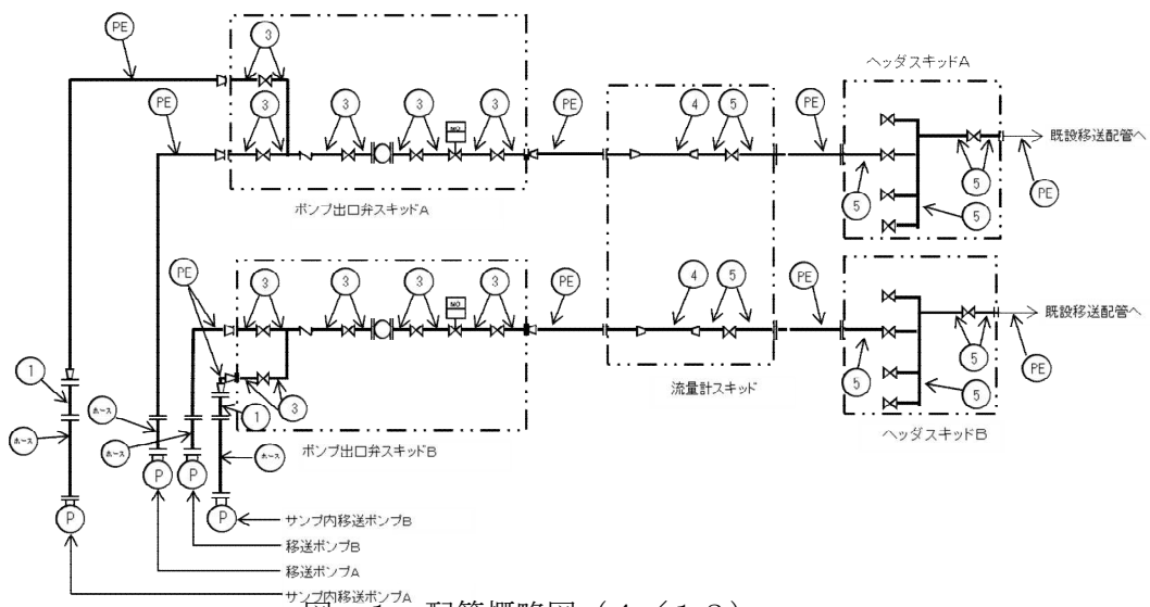
図ー1 配管概略図 (4 / 12)
