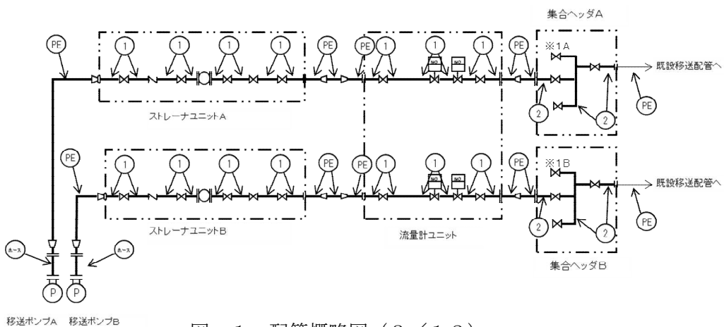
図ー1 配管概略図 (3 / 12)
