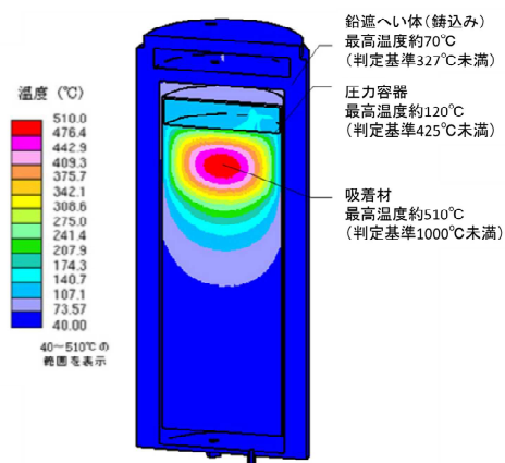
図2 吸着塔A型の温度分布
