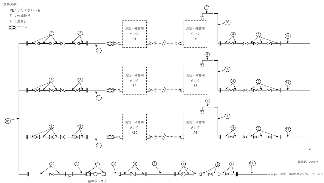
図－３ 配管概略図（３／５） （測定・確認用設備）
