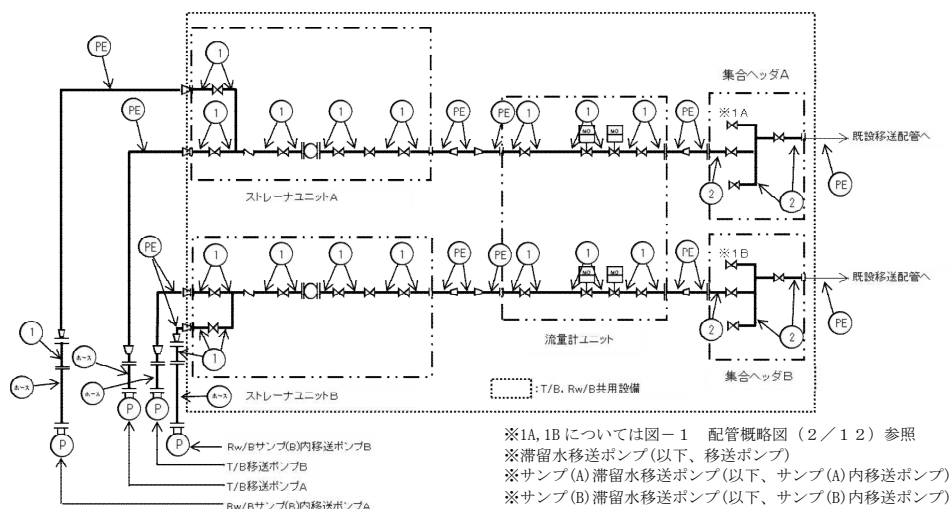
図－１ 配管概略図（１／１２）
