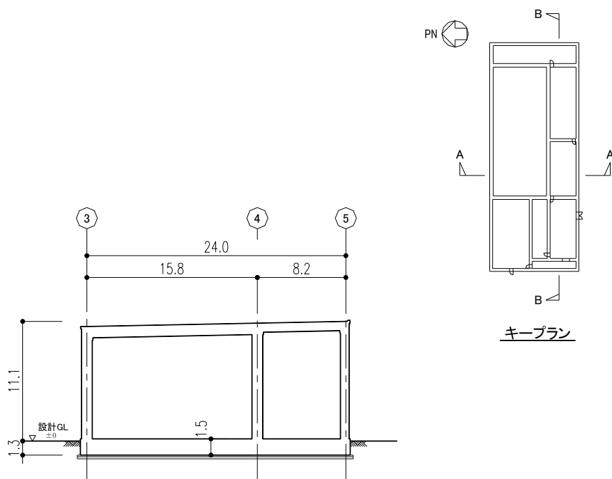
図ー3 スラッジ棟 A-A断面図 (NS 方向) (単位：m)
