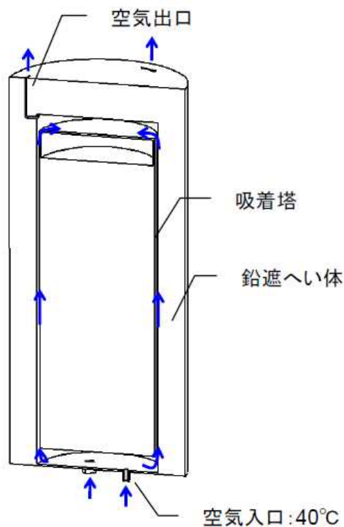
図－3 (TYPE-A) 同時吸着塔 解析モデル (概念図)
