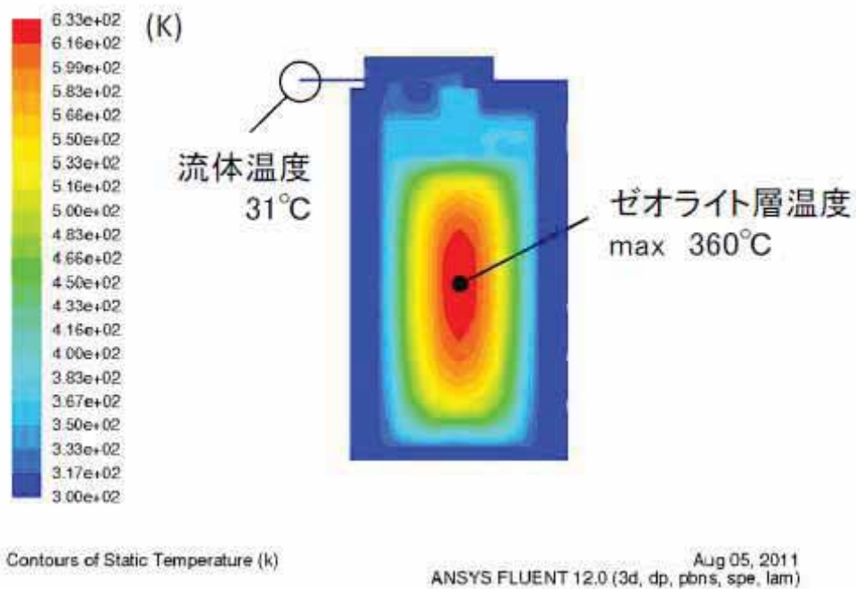
図－１ ３次元解析計算によるセシウム吸着装置吸着塔の温度分布
