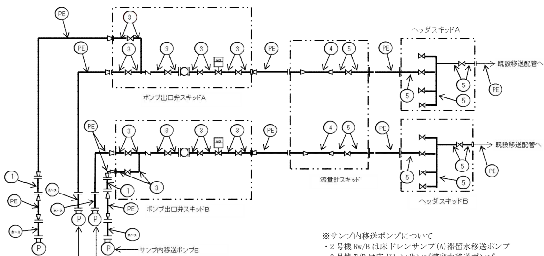
図－1 配管概略図 (6 / 12) (2号機 Rw/B 3号機 T/B, Rw/B)
