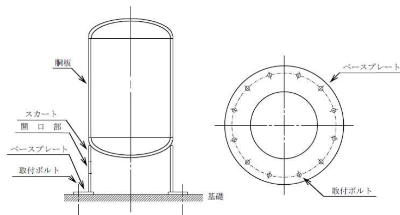
図－１ ろ過フィルタ・吸着塔Ａ型概要図
