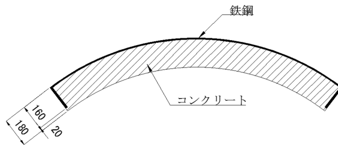
図－８－２ セグメント標準断面図（円周方向）（鉄鋼コンクリート造）
