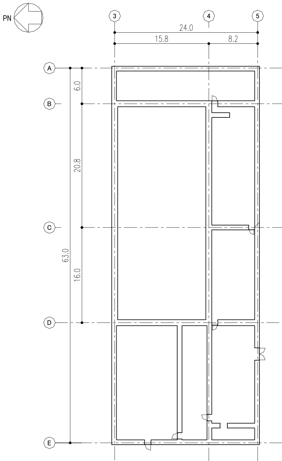
図ー１ スラッジ棟 建屋平面図（設計 G.L. +0.2）（単位：m）
