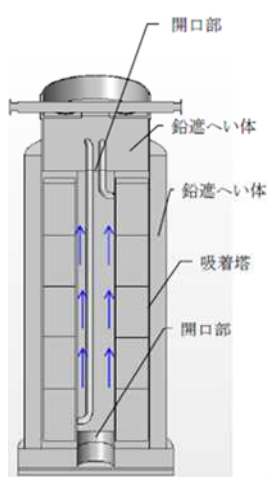
図3 吸着塔B型解析モデル（概念図）
