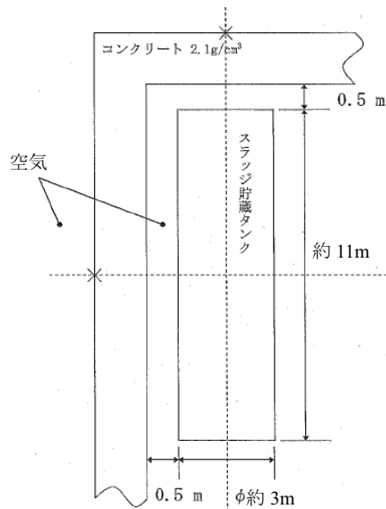
図ー１ 廃スラッジ一時保管施設 建屋外壁評価モデル
