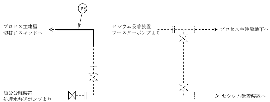
図ー1 配管概略図（5／5）
