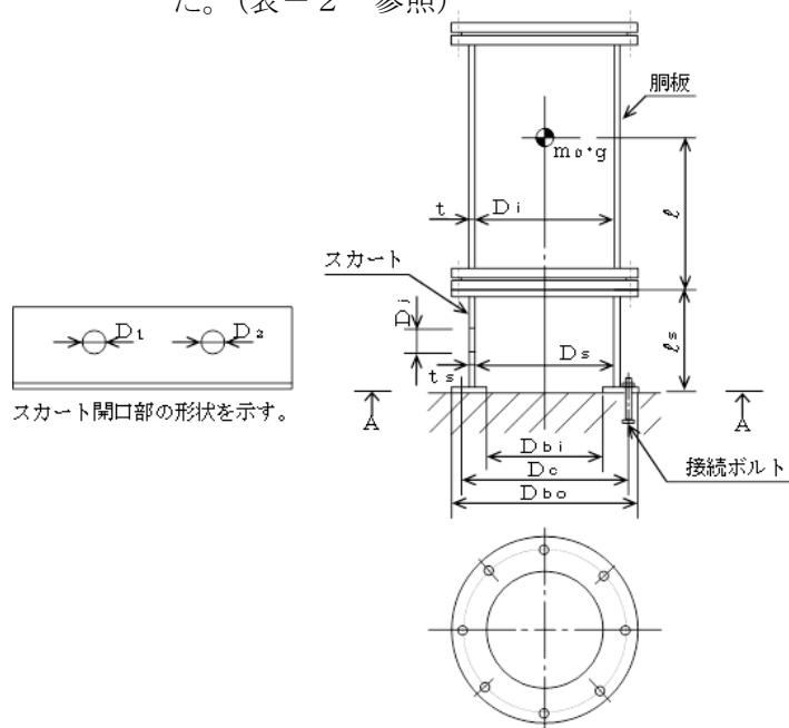
A~A矢视图
