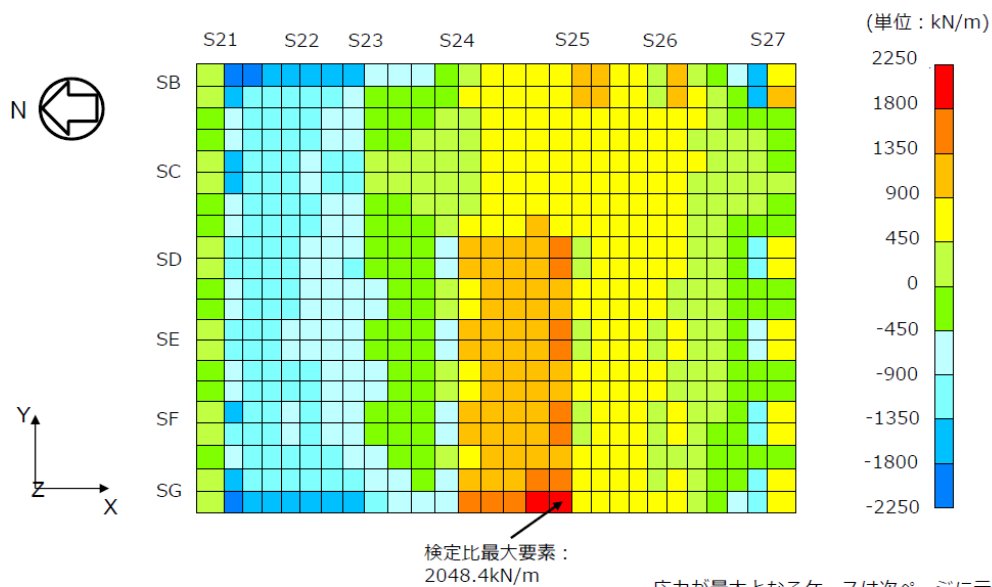
応力コンター (NS方向せん断力) 検定比最大値発生荷重ケース: Ss-1+NS-UD(A)
