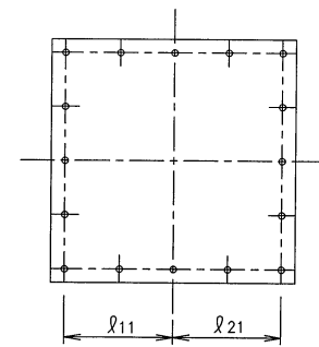
A-A矢視図
