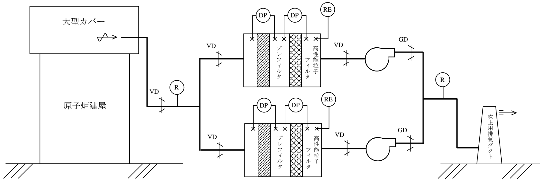
図 5-4 大型カバー換気設備系統図
