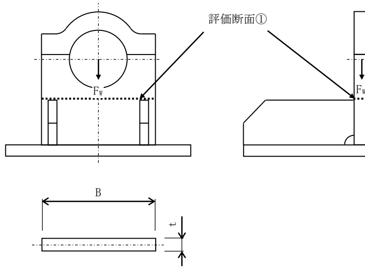
評価断面図
