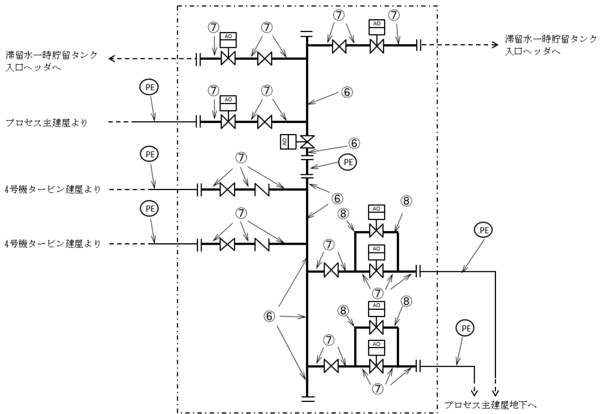
図-1 配管概略図 (3 / 5)
