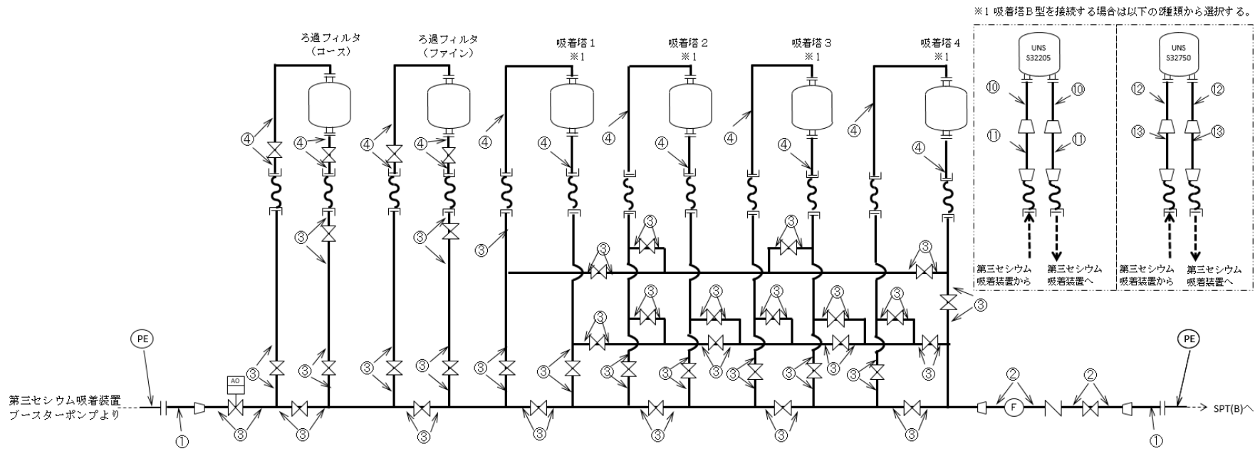
図-1 配管概略図 (2 / 5)
