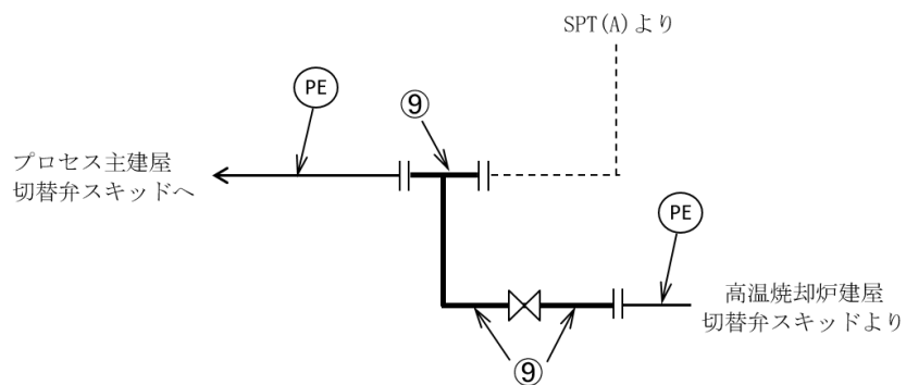
図-1 配管概略図 (4 / 5)
