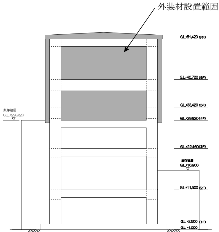
南側立面図
