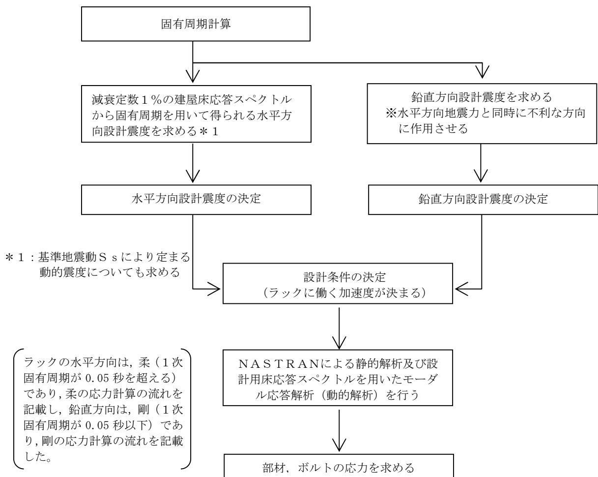
図1-1 ラックの耐震評価フロー
