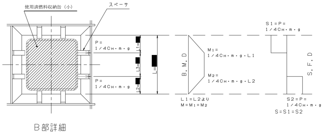
図 8 - 3 スペーサおよびスペーサ下部支持部材の作用荷重 (2/2)
