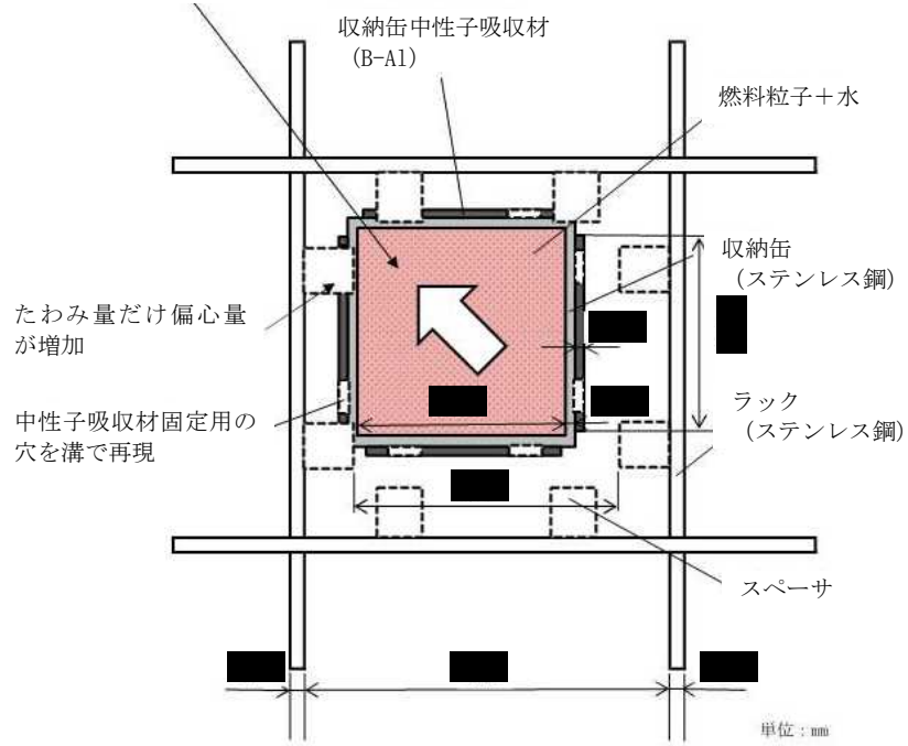
図-2 収納缶のラックセル内偏心配置
