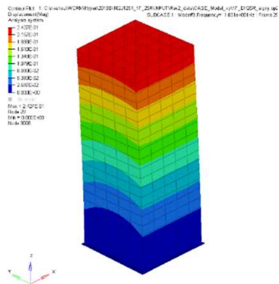
図 3-5 振動モード (3次モード)
