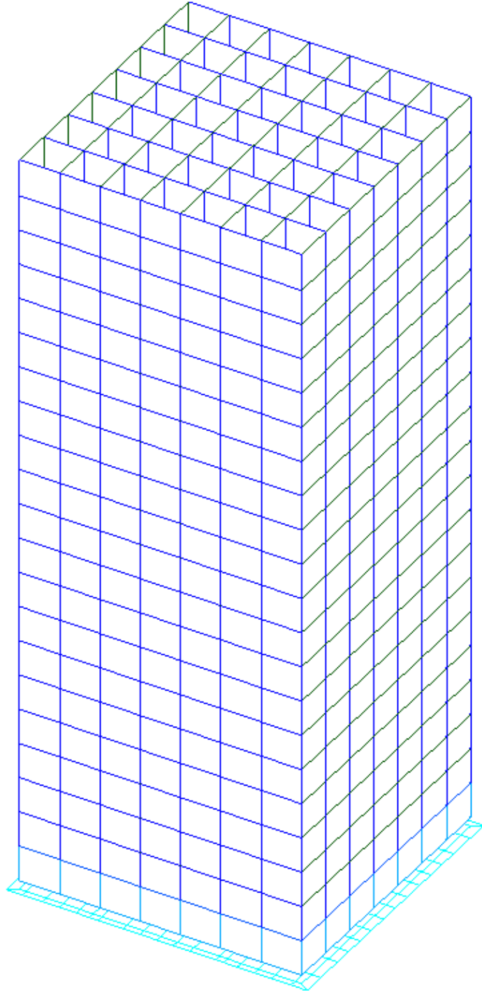
図2-1 使用済燃料貯蔵ラック（49体）計算モデル
