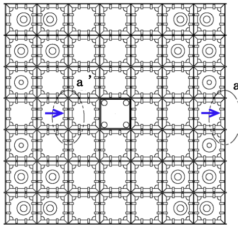
図 8-1 使用済燃料貯蔵ラック（49 体）上面図
