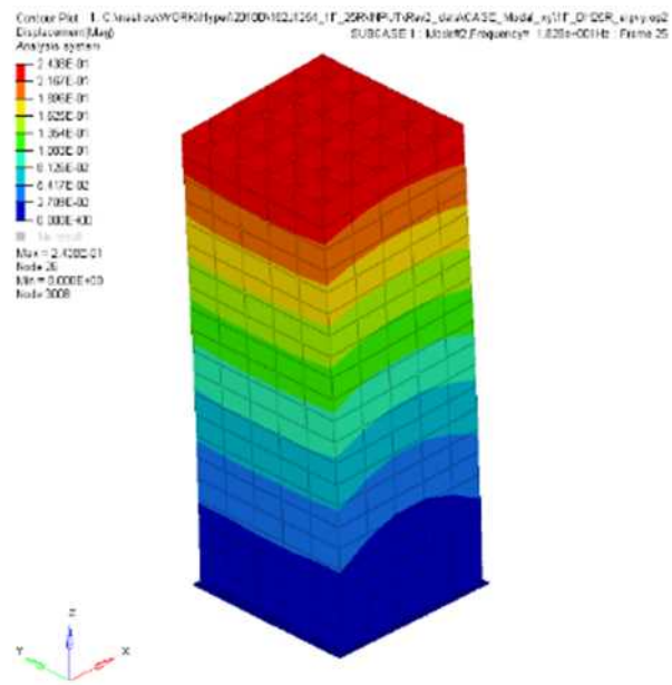
図 3-4 振動モード (2次モード)
