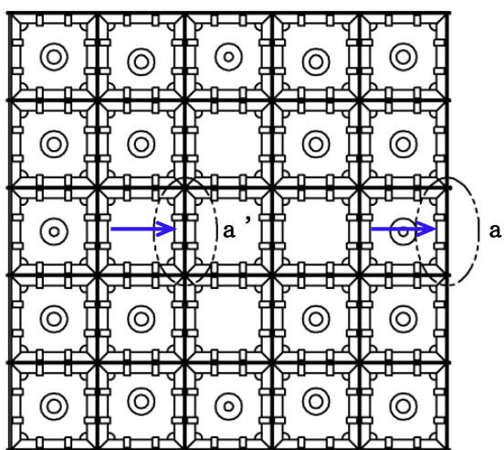
図3-9 使用済燃料貯蔵ラック（25 体）上面図
