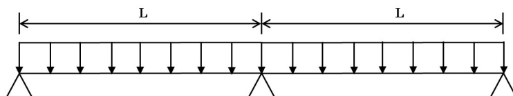
図-2 等分布荷重 3点支持はりモデル
