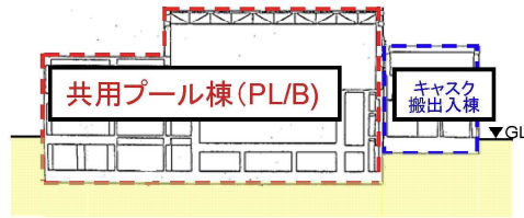
共用プール棟 (PL/B) ・ キャスク搬出入棟 NS方向断面図
