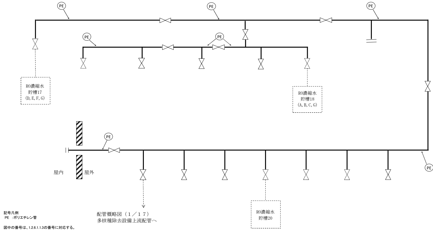
図-1 配管概略図 (2 / 17)
