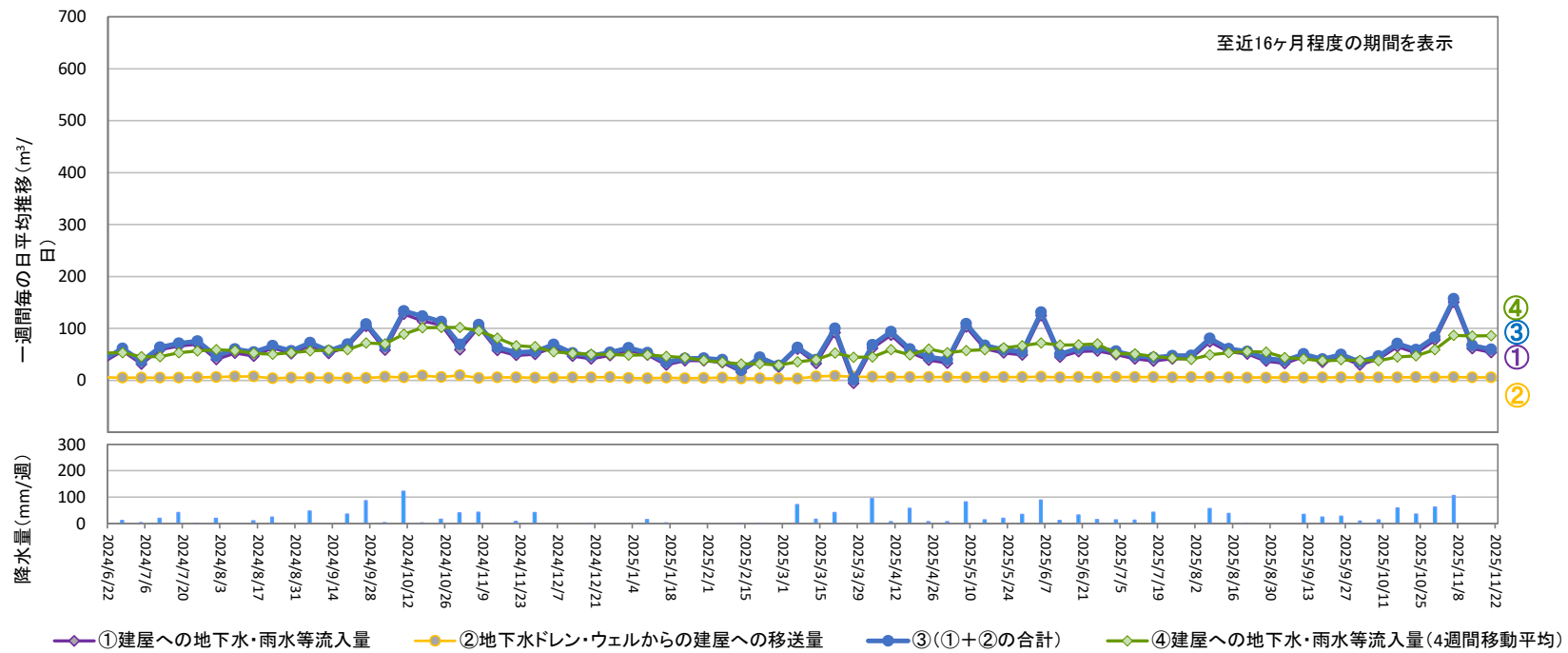
地下水ドレンからタービン建屋への移送量 ( 2025年11月13日 ～ 2025年11月19日 ) [m³/日]
