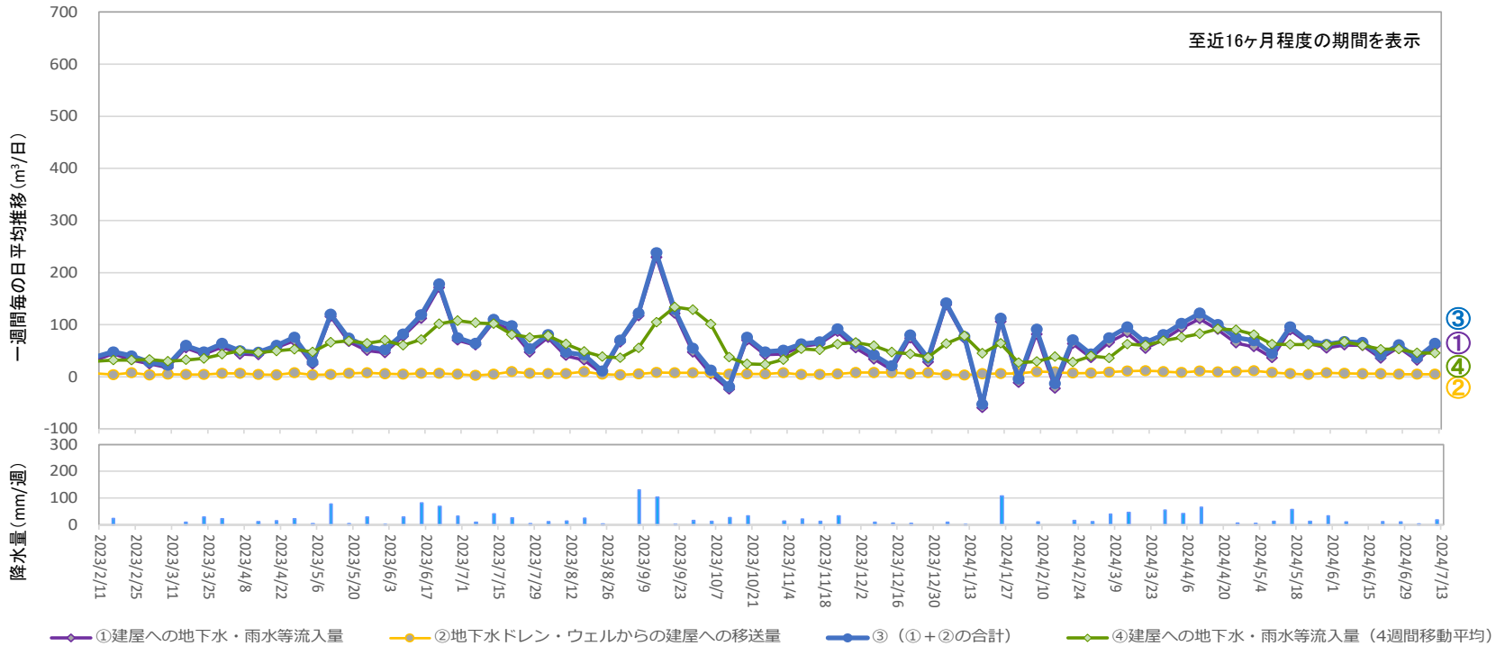
地下水ドレンからタービン建屋への移送量 ( 2024年7月4日 ~ 2024年7月10日 )
