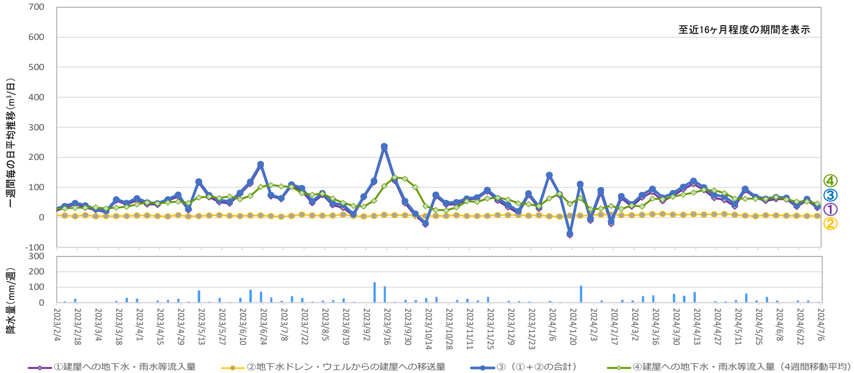
地下水ドレンからタービン建屋への移送量 ( 2024年6月27日 ~ 2024年7月3日 )
