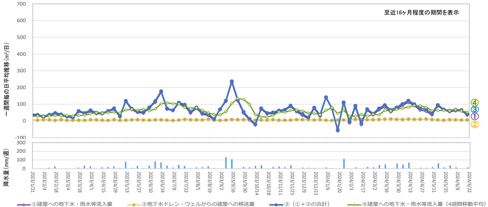
地下水ドレンからタービン建屋への移送量 ( 2024年6月13日 ~ 2024年6月19日 )
