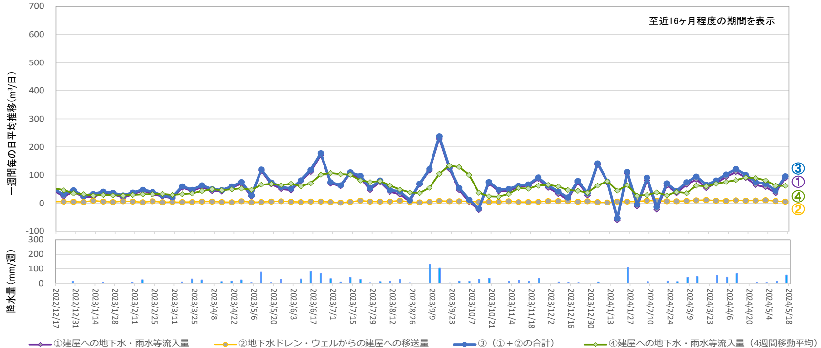
地下水ドレンからタービン建屋への移送量 ( 2024年5月9日 ~ 2024年5月15日 )
