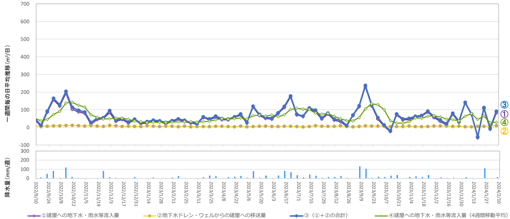
地下水ドレンからタービン建屋への移送量 ( 2024年2月1日 ~ 2024年2月7日 )
