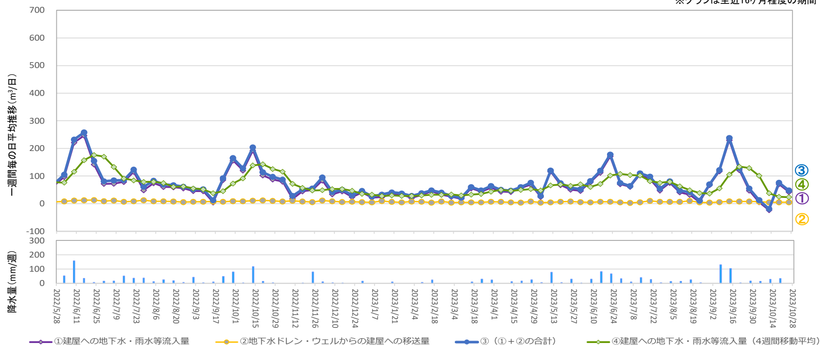
地下水ドレンからタービン建屋への移送量 ( 2023年10月19日 ~ 2023年10月25日 )
