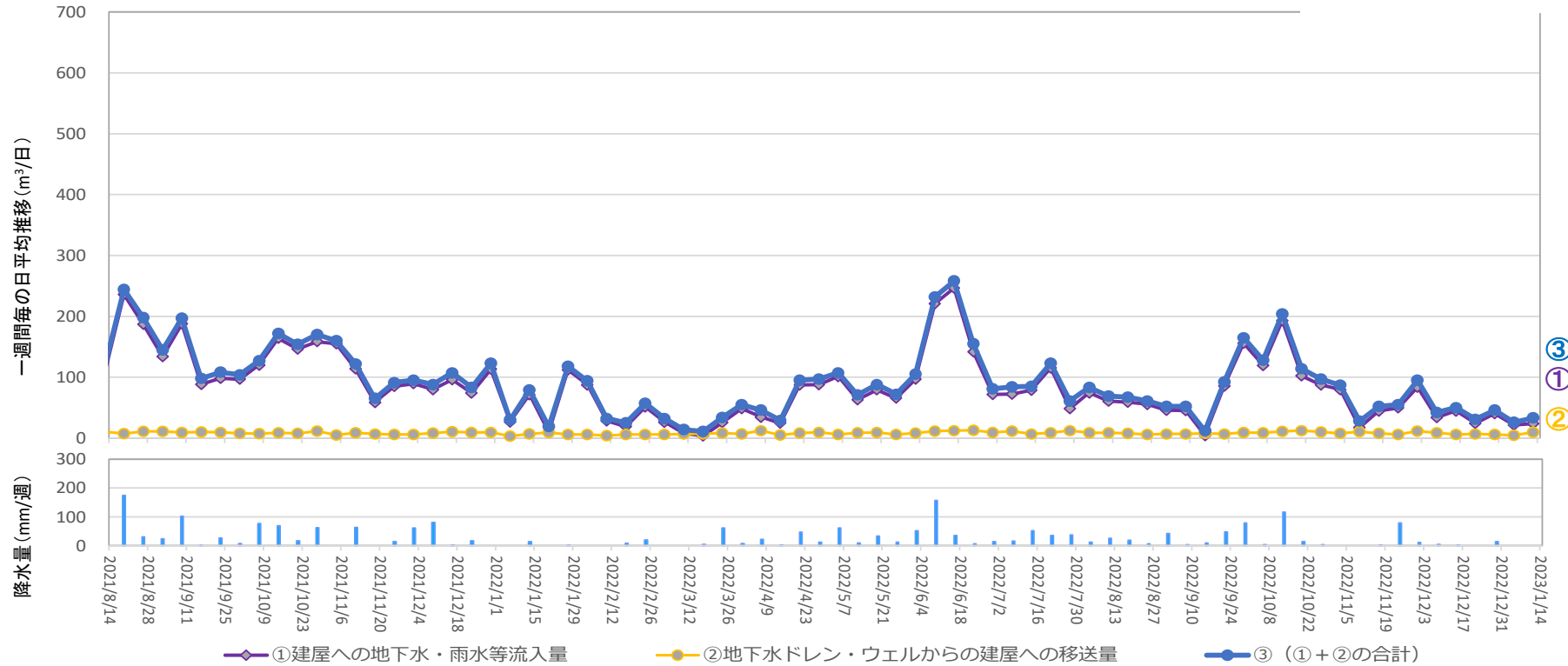
地下水ドレンからタービン建屋への移送量 ( 2023年1月5日 ~ 2023年1月11日 )
