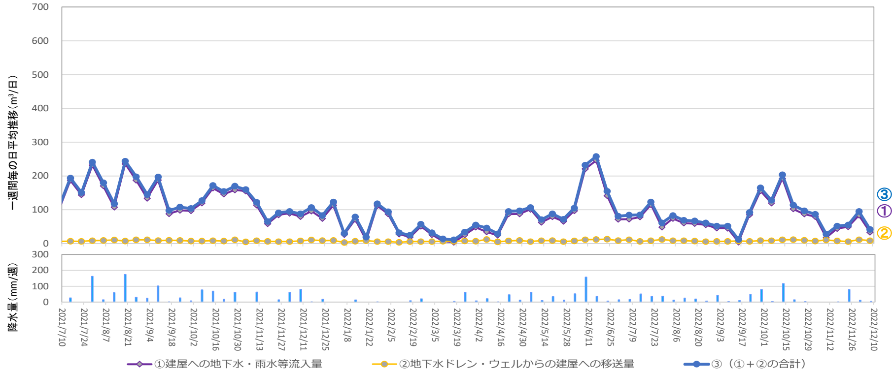
地下水ドレンからタービン建屋への移送量 ( 2022年12月1日 ~ 2022年12月7日 )
