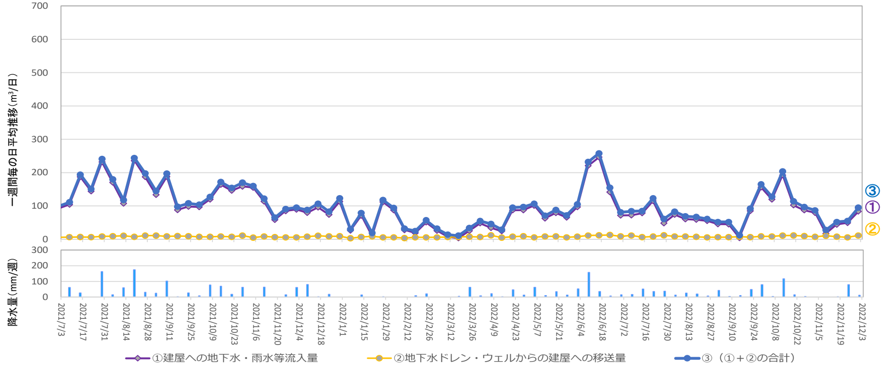
地下水ドレンからタービン建屋への移送量 ( 2022年11月24日 ~ 2022年11月30日 )
