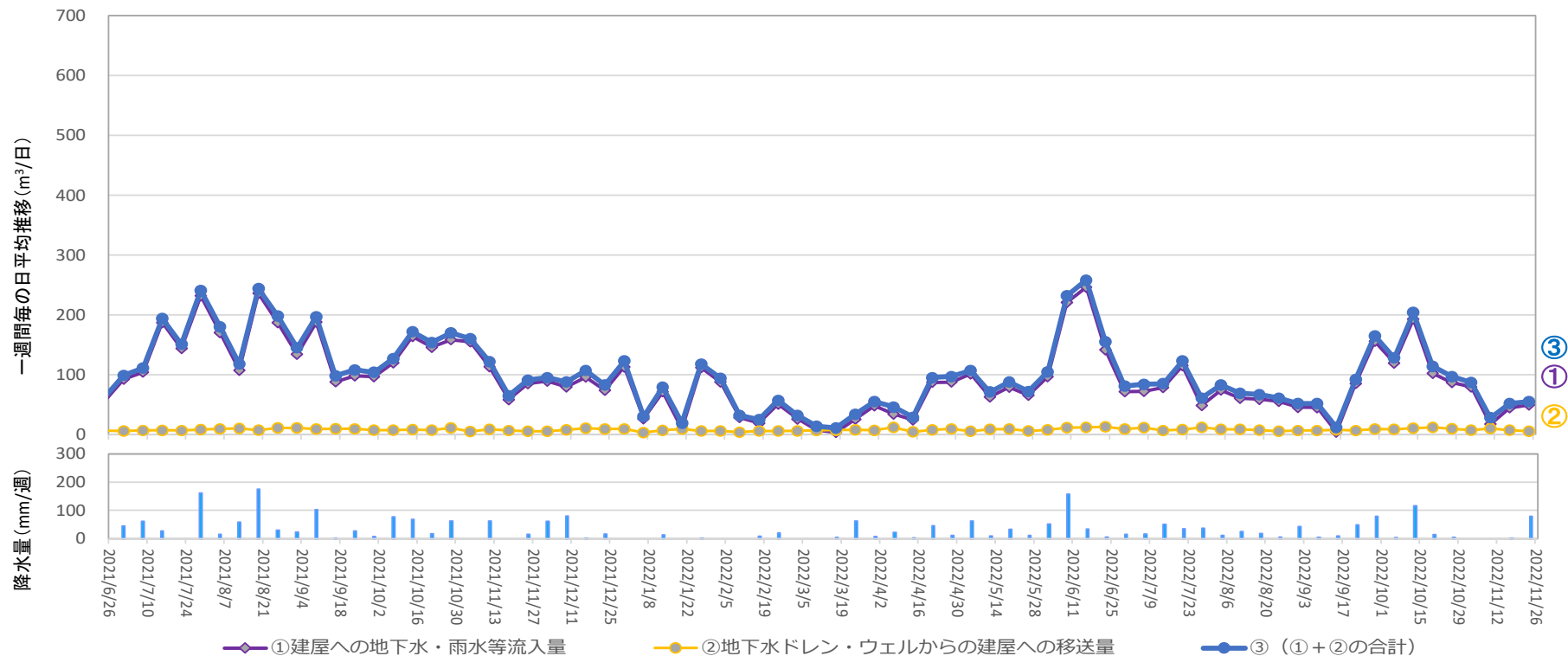
地下水ドレンからタービン建屋への移送量 ( 2022年11月17日 ~ 2022年11月23日 )
