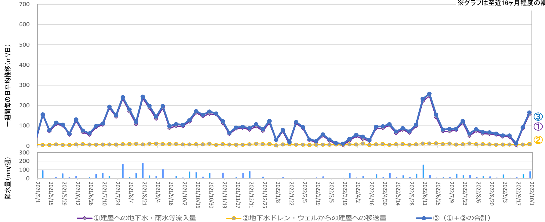
地下水ドレンからタービン建屋への移送量 ( 2022年9月22日 ~ 2022年9月28日 )
