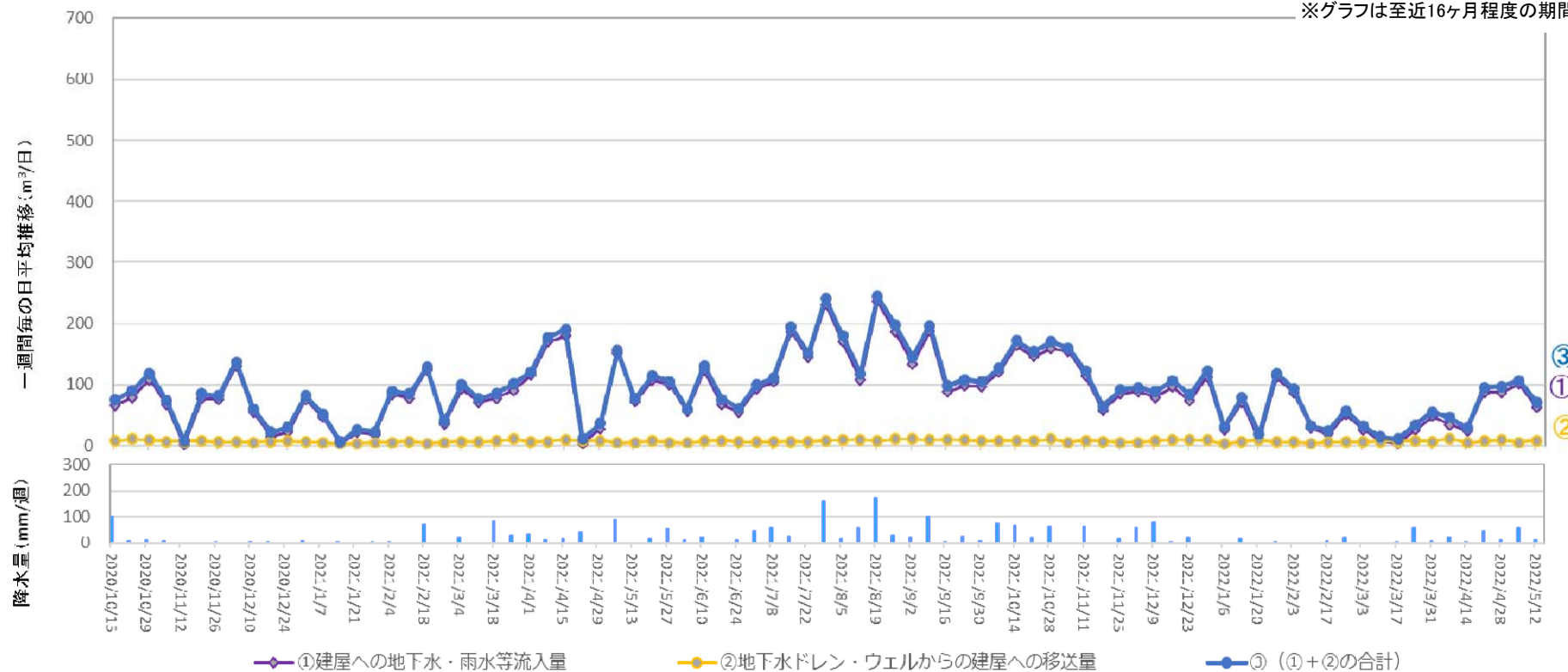
地下水ドレンからタービン建屋への移送量 ( 2022年5月5日 ~ 2022年5月11日 )
