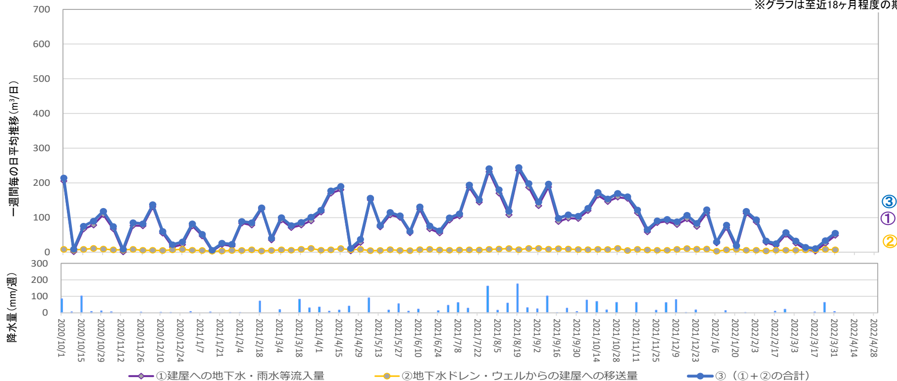
地下水ドレンからタービン建屋への移送量 ( 2022年3月24日 ~ 2022年3月30日 )
