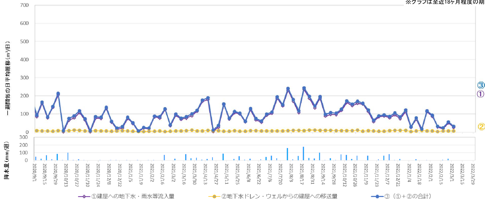
地下水ドレンからタービン建屋への移送量 ( 2022年2月24日 ~ 2022年3月2日 )
