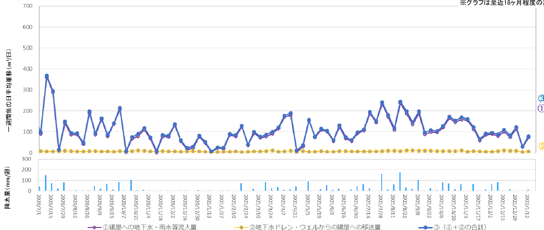
地下水ドレンからタービン建屋への移送量 ( 2022年1月6日 ~ 2022年1月12日 )
