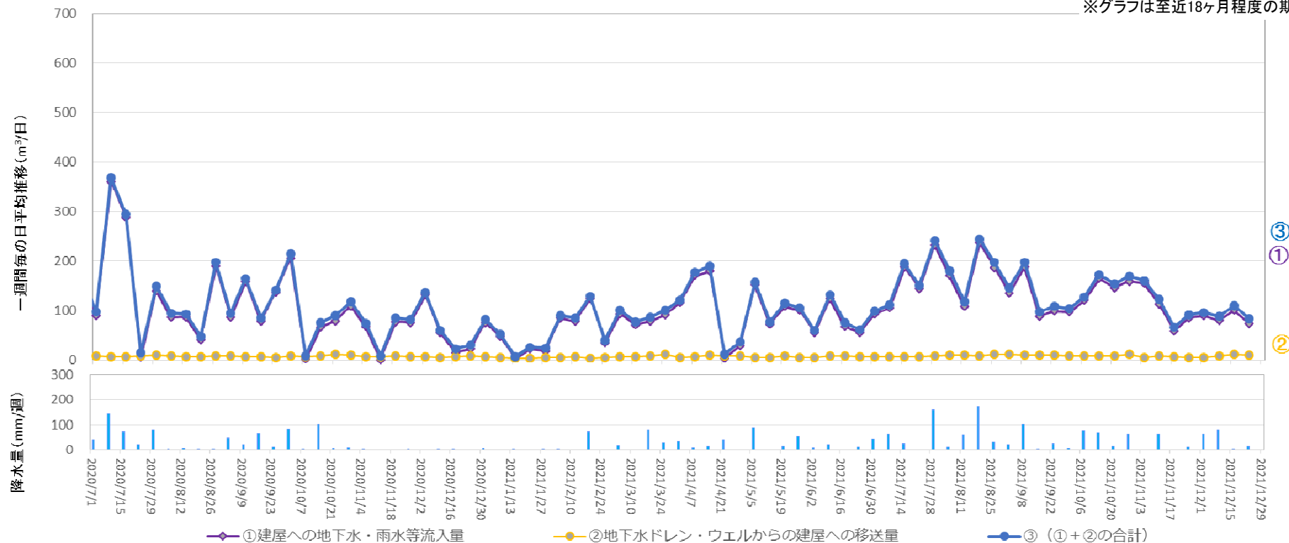
地下水ドレンからタービン建屋への移送量 (2021年12月16日 ~ 2021年12月22日)
