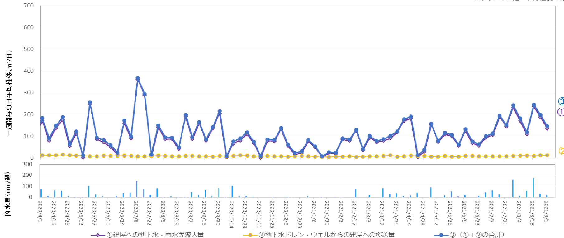
地下水ドレンからタービン建屋への移送量 ( 2021年8月26日 ~ 2021年9月1日 )
