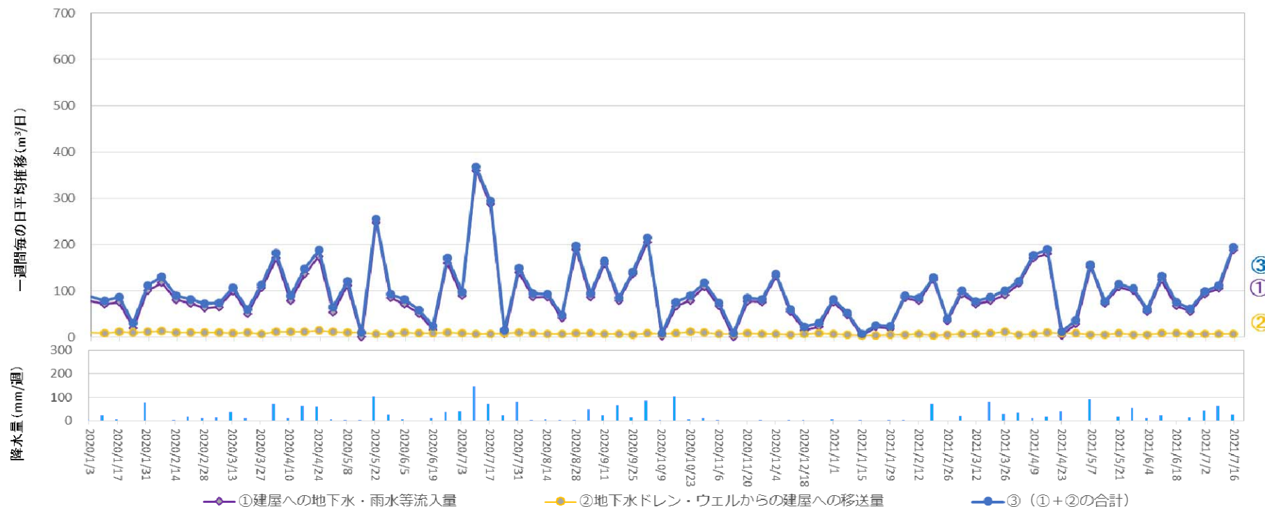
地下水ドレンからタービン建屋への移送量 ( 2021年7月8日 ~ 2021年7月14日 )
