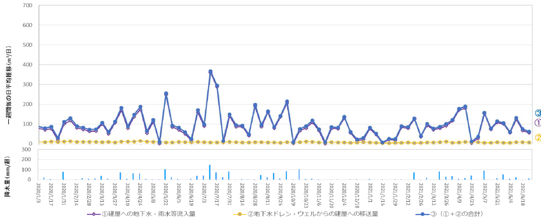
地下水ドレンからタービン建屋への移送量 ( 2021年6月17日 ~ 2021年6月23日 )
