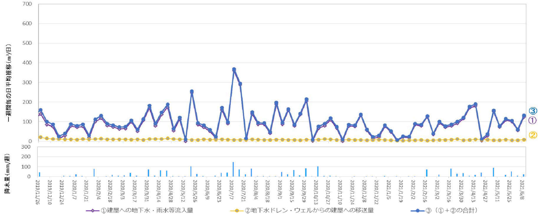
地下水ドレンからタービン建屋への移送量 ( 2021年6月3日 ~ 2021年6月9日 )
