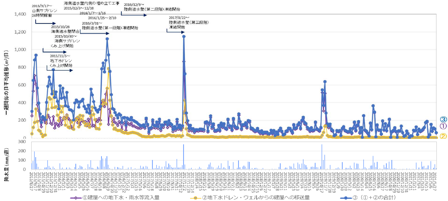
① 建屋への地下水・雨水等流入量 ② 地下水ドレン・ウェルからの建屋への移送量 ③ (①+②の合計)
