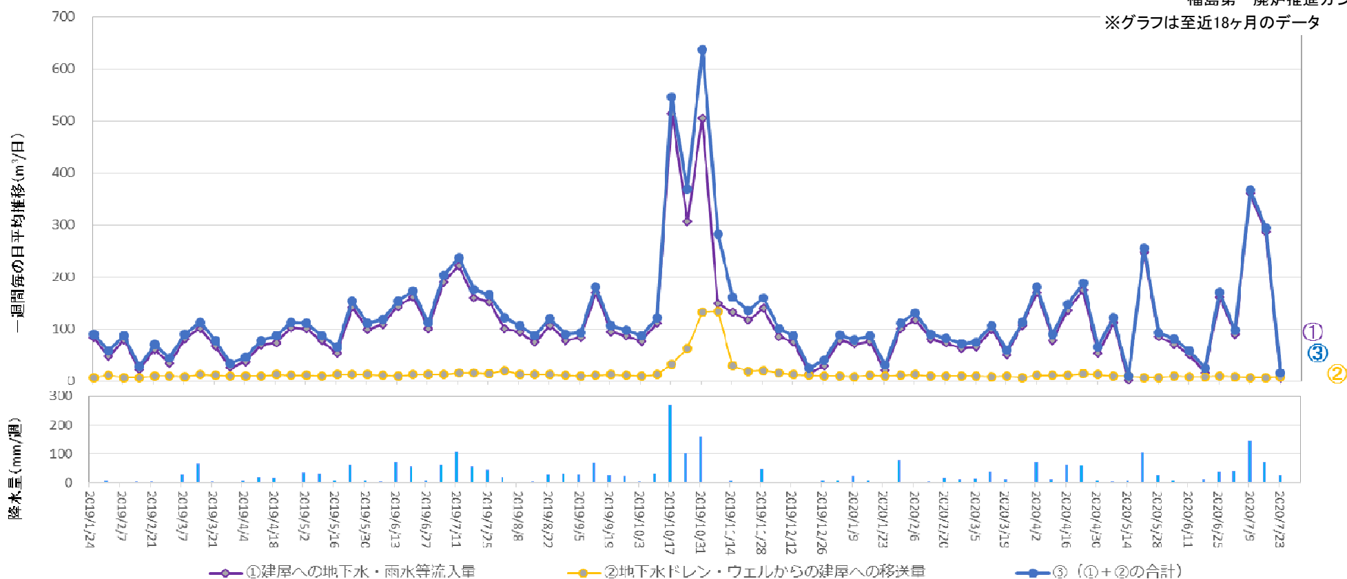
地下水ドレンからタービン建屋への移送量 (2020年7月16日 ~ 2020年7月22日)
