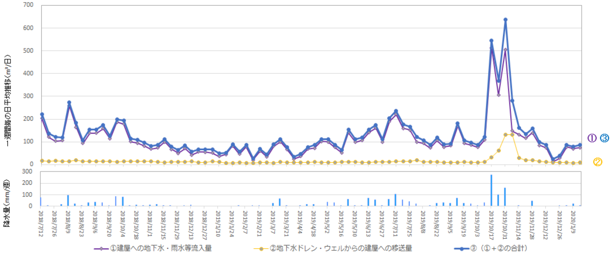
地下水ドレンからタービン建屋への移送量 ( 2020年1月9日 ~ 2020年1月15日 )
