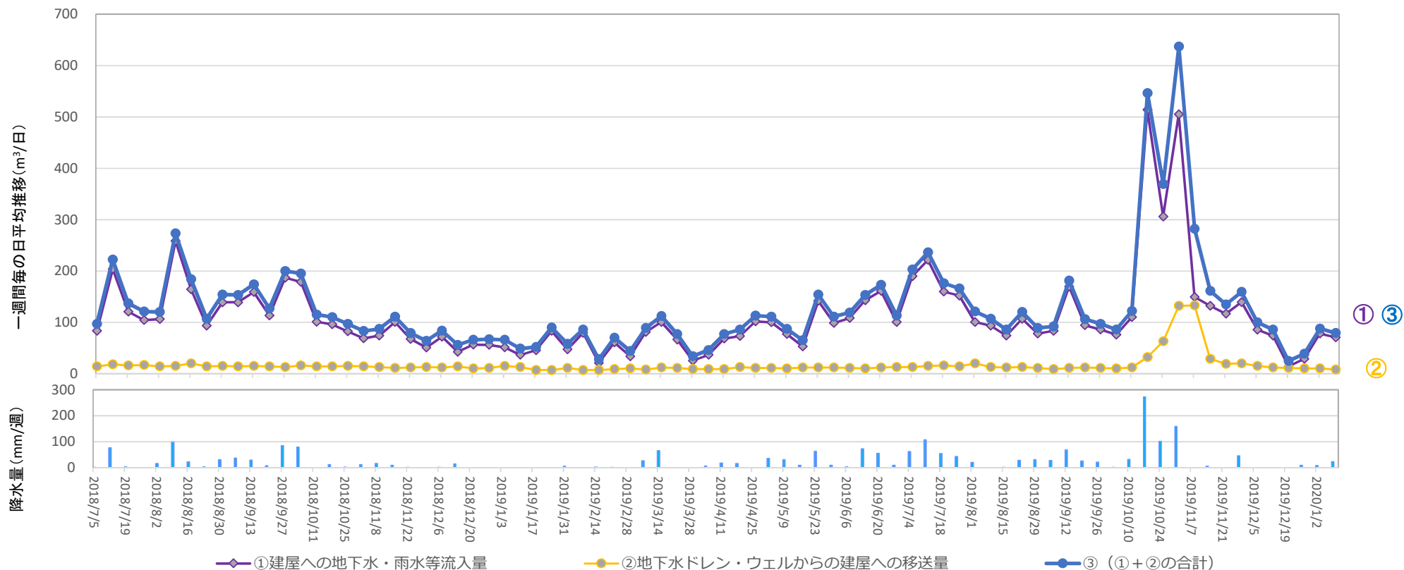
地下水ドレンからタービン建屋への移送量 ( 2020年1月2日 ~ 2020年1月8日 )
