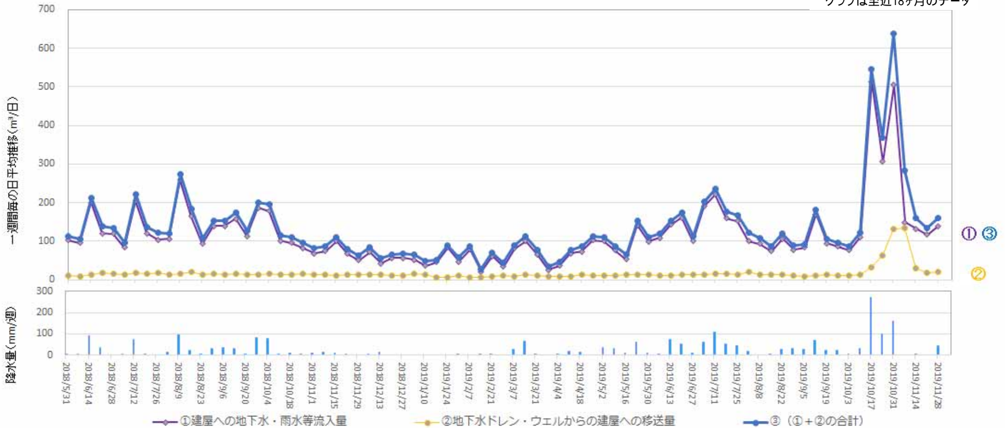
地下水ドレンからタービン建屋への移送量 (2019年11月21日 ~ 2019年11月27日)
