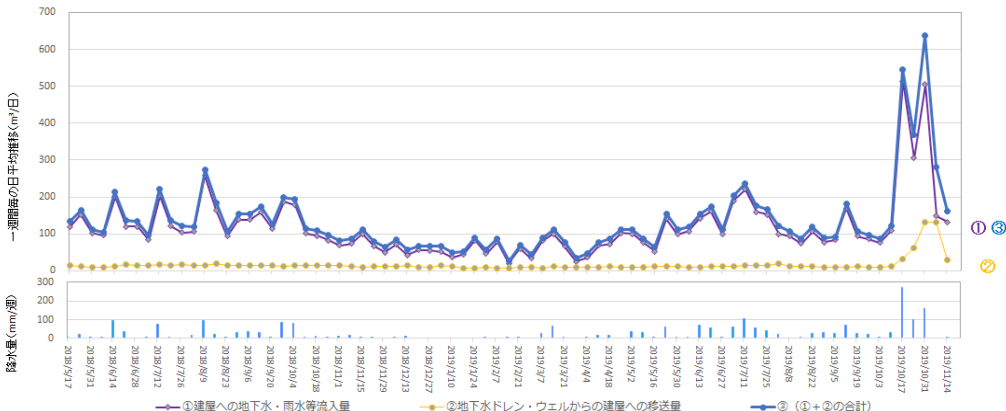
地下水ドレンからタービン建屋への移送量 (2019年11月7日 ~ 2019年11月13日)
