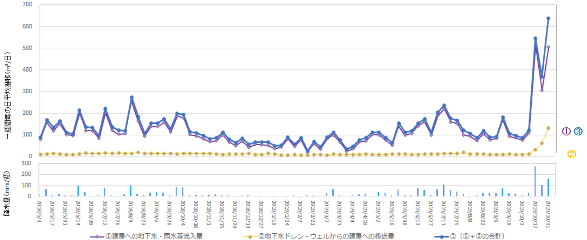
地下水ドレンからタービン建屋への移送量 (2019年10月24日 ~ 2019年10月30日)
