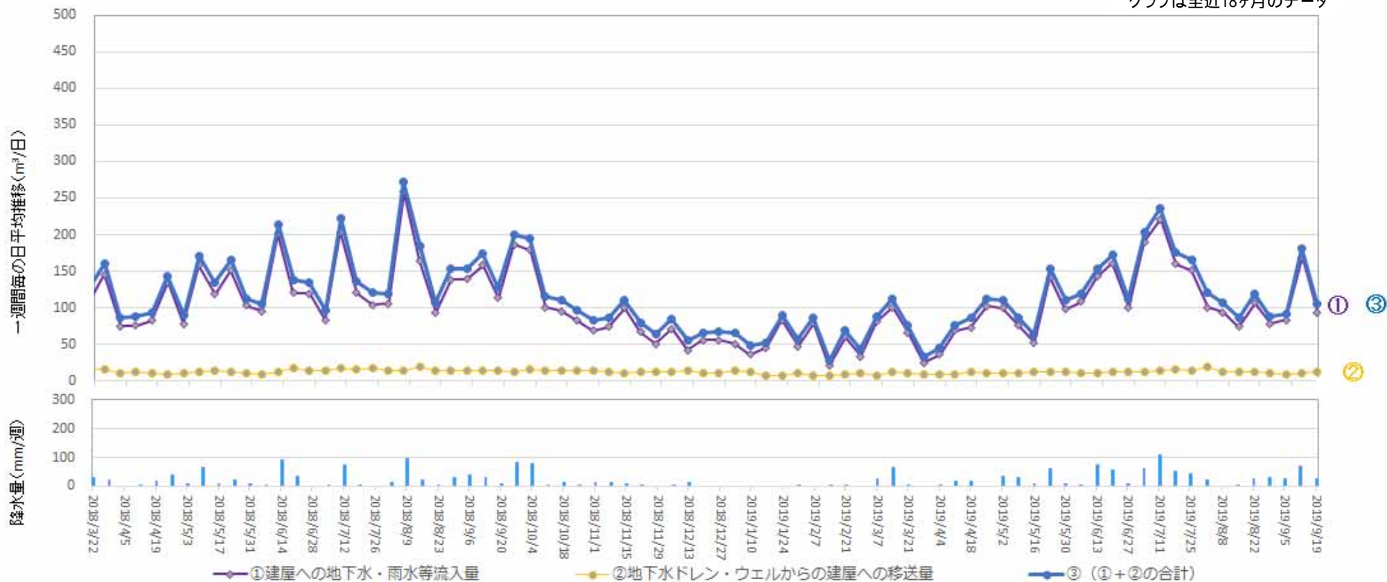
地下水ドレンからタービン建屋への移送量 (2019年9月12日 ~ 2019年9月18日)
