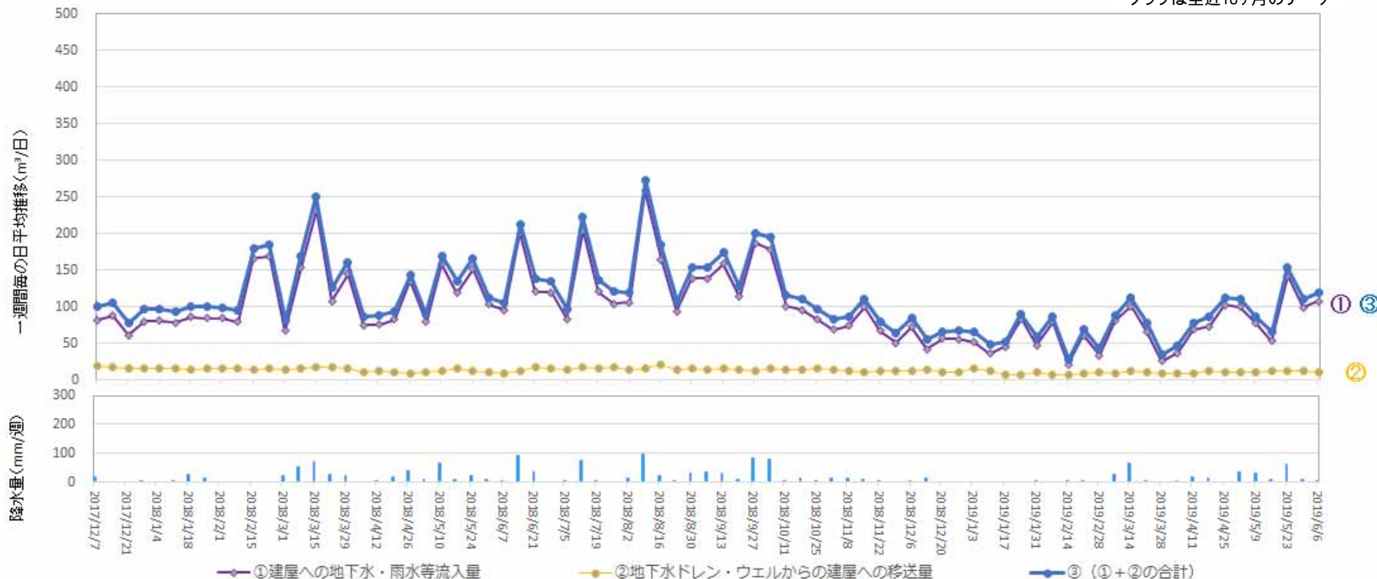
地下水ドレンからタービン建屋への移送量 ( 2019年5月30日 ~ 2019年6月5日 )
