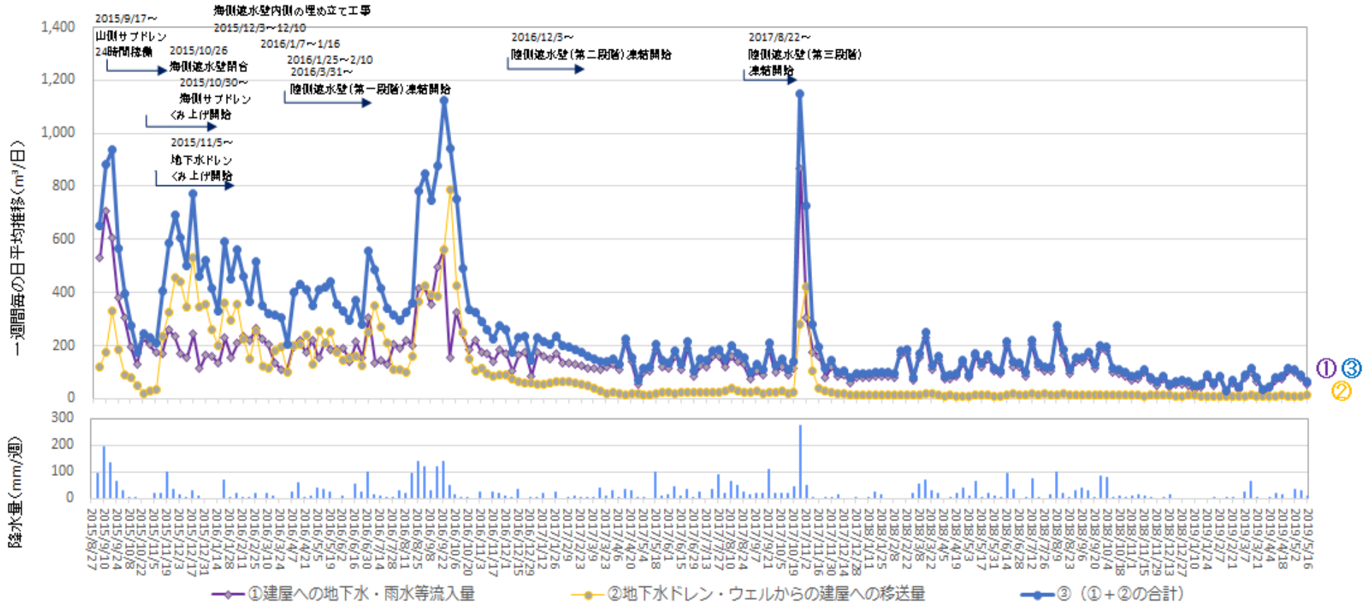
地下水ドレンからタービン建屋への移送量 ( 2019年5月9日 ~ 2019年5月15日 )
