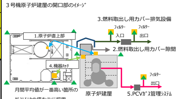
3号機原子炉建屋の開口部のイメージ 月間平均値が一番高い箇所のダストモニタの値を②に採用 ダスト測定箇所 ▲ダストモニタ ■フィルター
