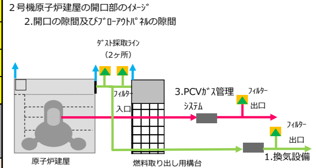
2号機原子炉建屋の開口部のイメージ 2. 開口の隙間及びBOPの隙間 ダスト採取ライン(2ヶ所) フィルター入口 原子炉建屋 燃料取り出し用構台 3. PCVガス管理システム フィルター出口 1. 換気設備 ダスト測定箇所 ▲ダストモニタ ■フィルター
