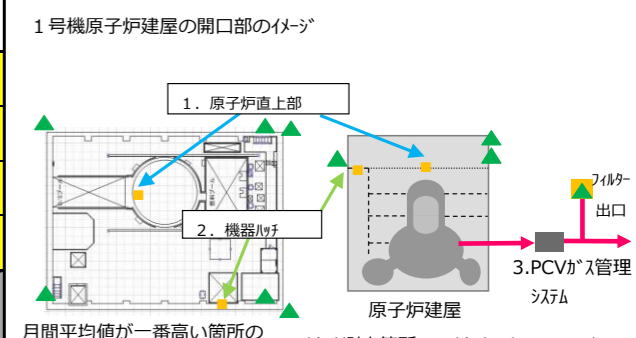
1号機原子炉建屋の開口部のイメージ 月間平均値が一番高い箇所のダスト測定箇所 ▲ダストモニタ ■フィルター ダストモニタの値を②に採用
