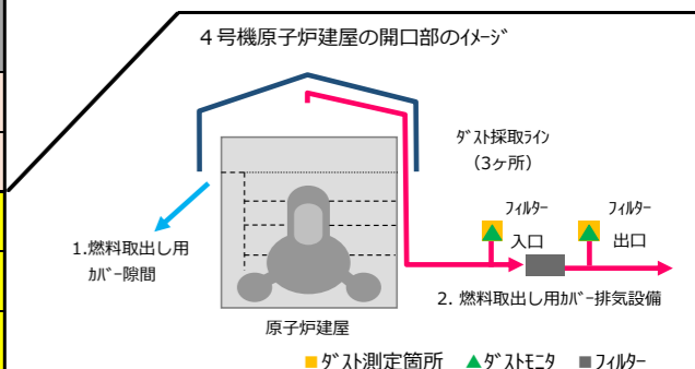
4号機原子炉建屋の開口部のイメージ ダスト採取ライン(3ヶ所) フィルター入口 1. 燃料取出し用カバー隙間 原子炉建屋 2. 燃料取出し用カバー排気設備 ダスト測定箇所 ▲ダストモニタ ■フィルター
